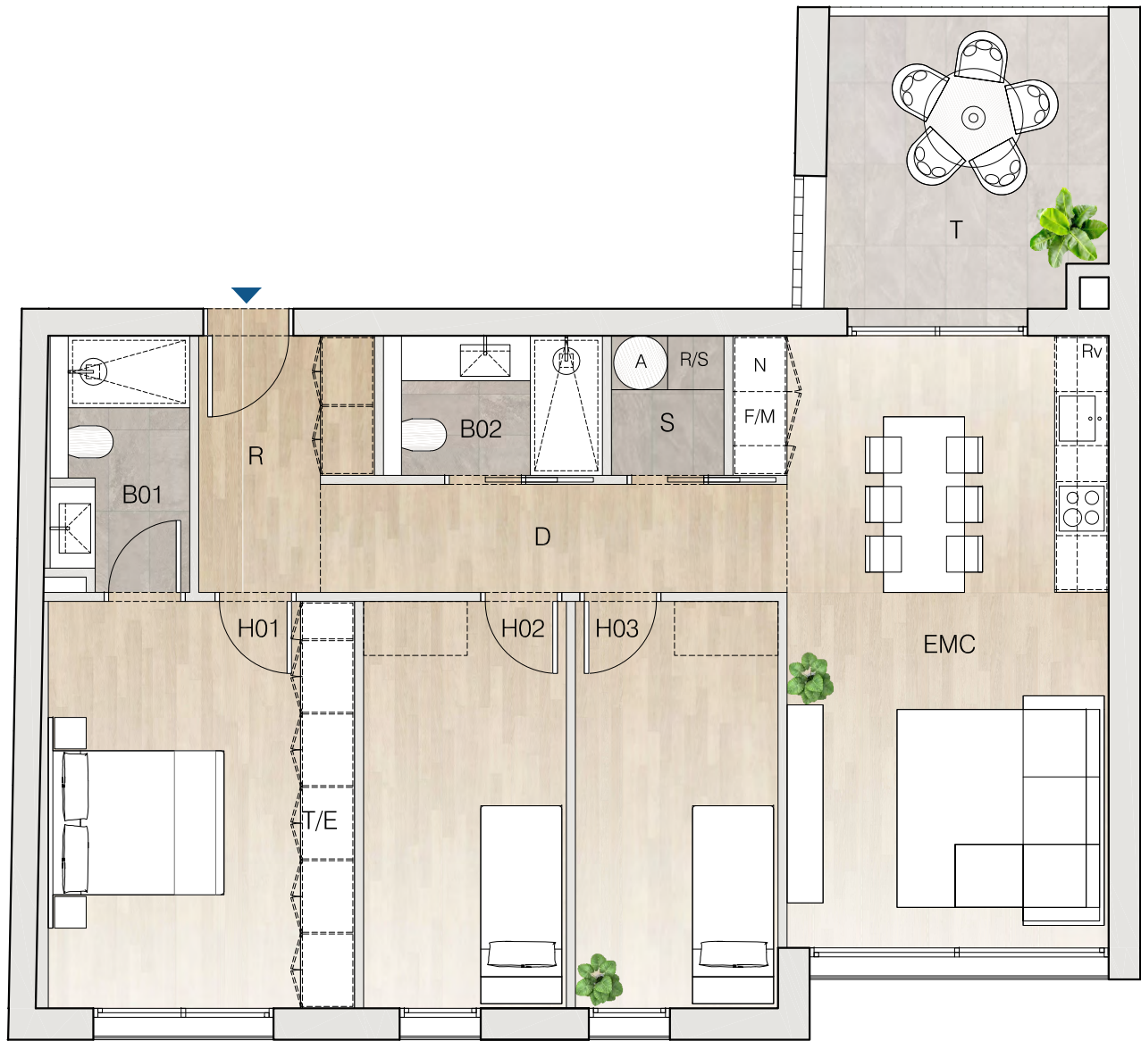
PLANTA HABITATGE 1 o -1 a (P1)
