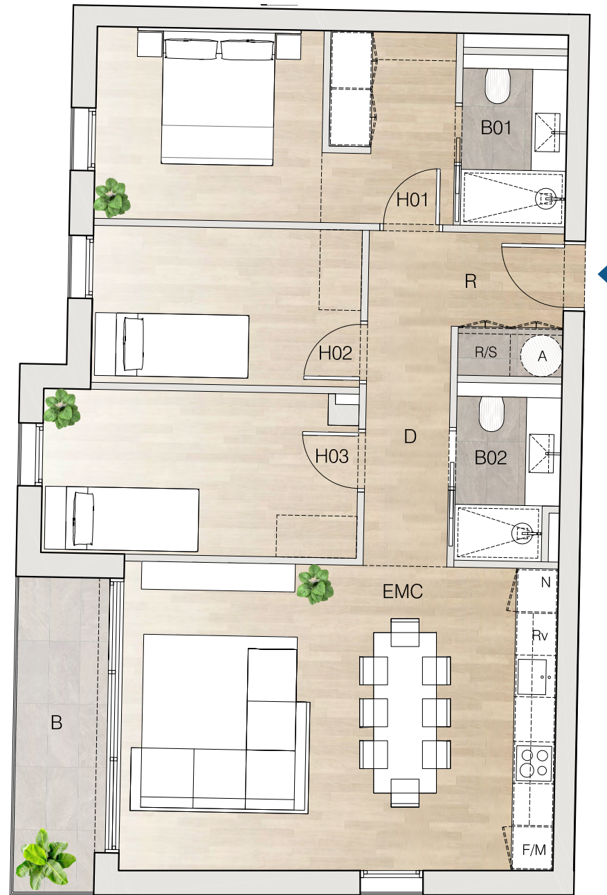
PLANTA HABITATGE 1º-2ª (P1)
