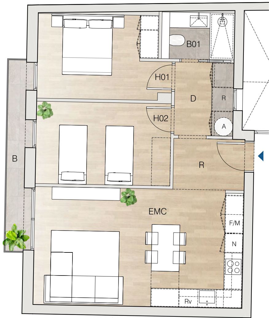
PLANTA HABITATGE 2º-3ª (P2)
