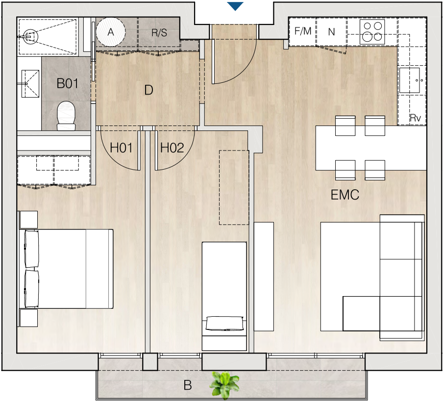
PLANTA HABITATGE 2º- 7ª (P2)
