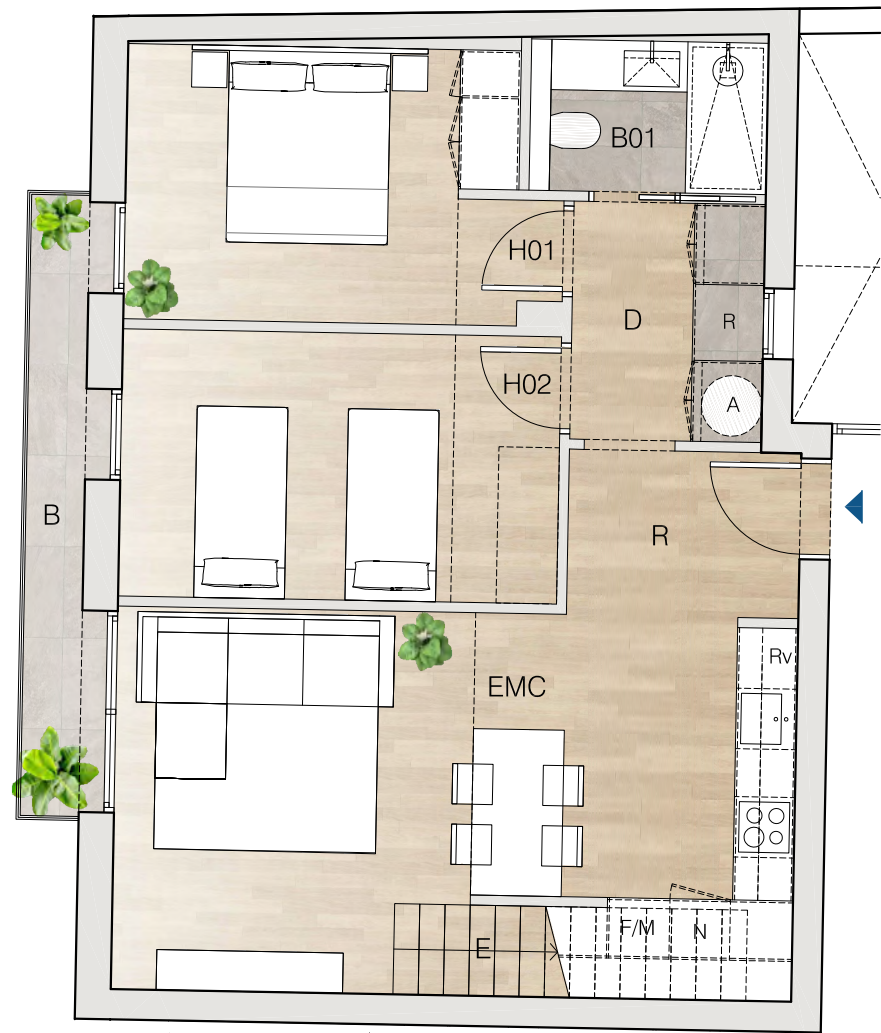
PLANTA HABITATGE 3º-3ª (P3)
