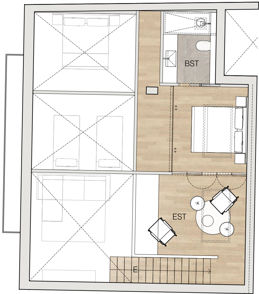
PLANTA HABITATGE ALTELL 3º-3ª (ST)
