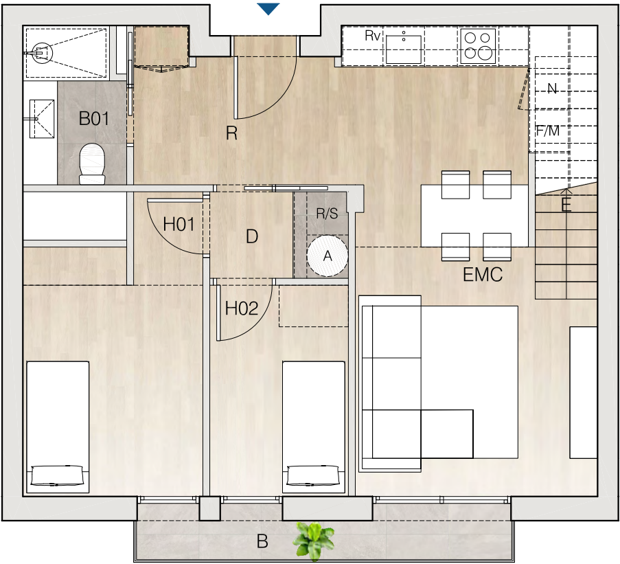
PLANTA HABITATGE 3º-7ª (P3)
