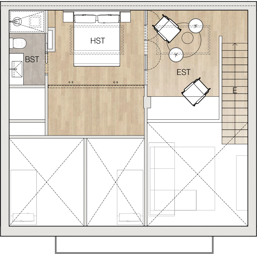
PLANTA HABITATGE ALTELL 3º-7ª (ST)
