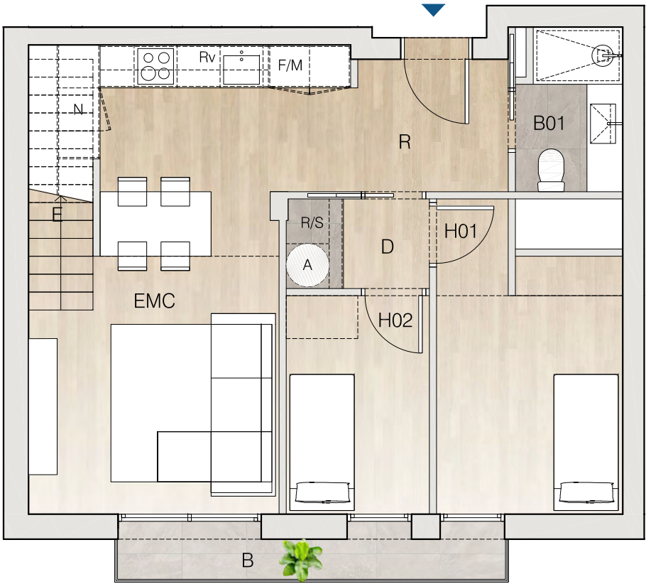
PLANTA HABITATGE 3º-8ª (P3)
